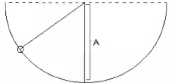
Circular pendulum.
